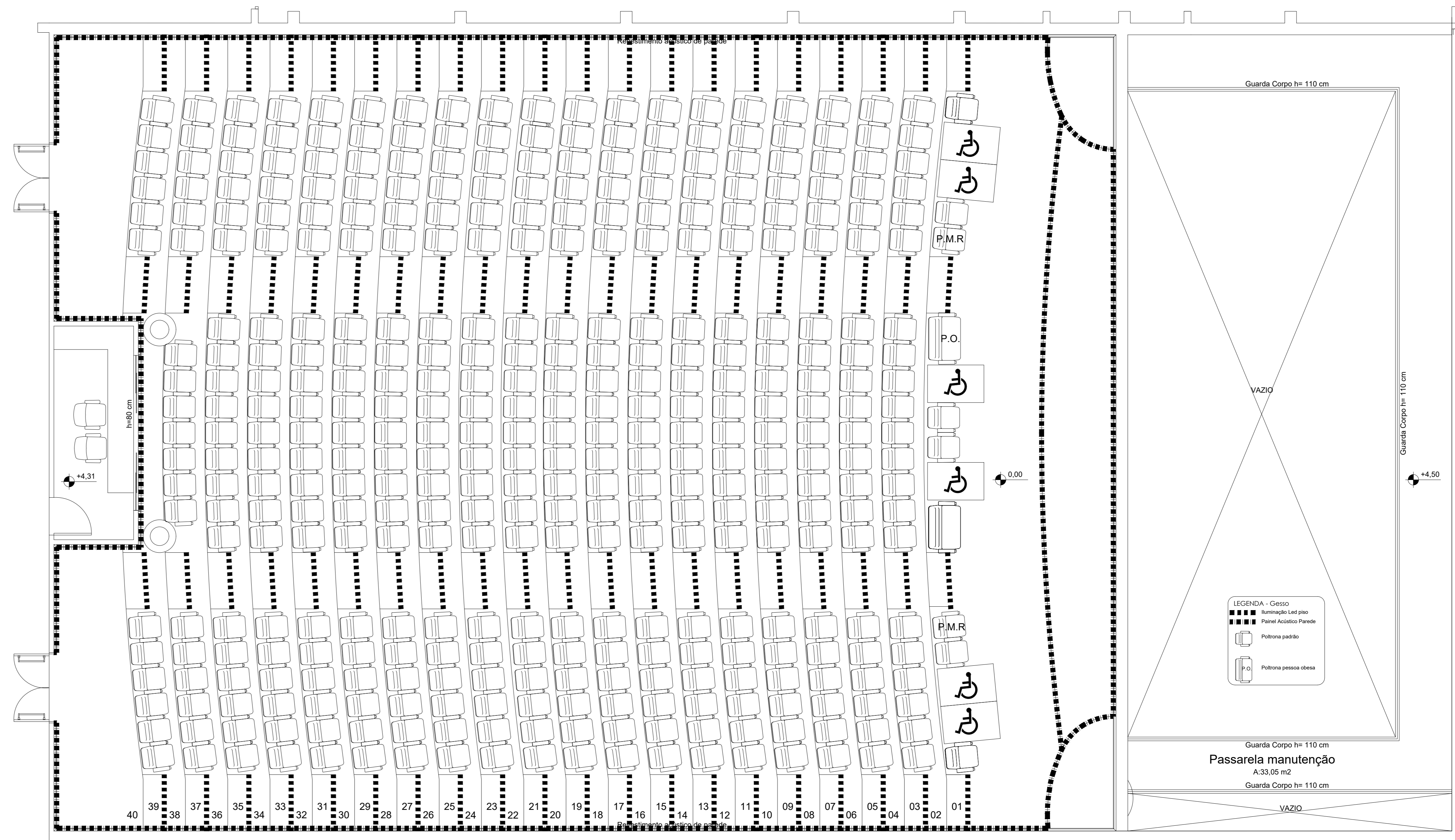
9 Layout Platéia e Iluminação Led piso Escala 1:50
