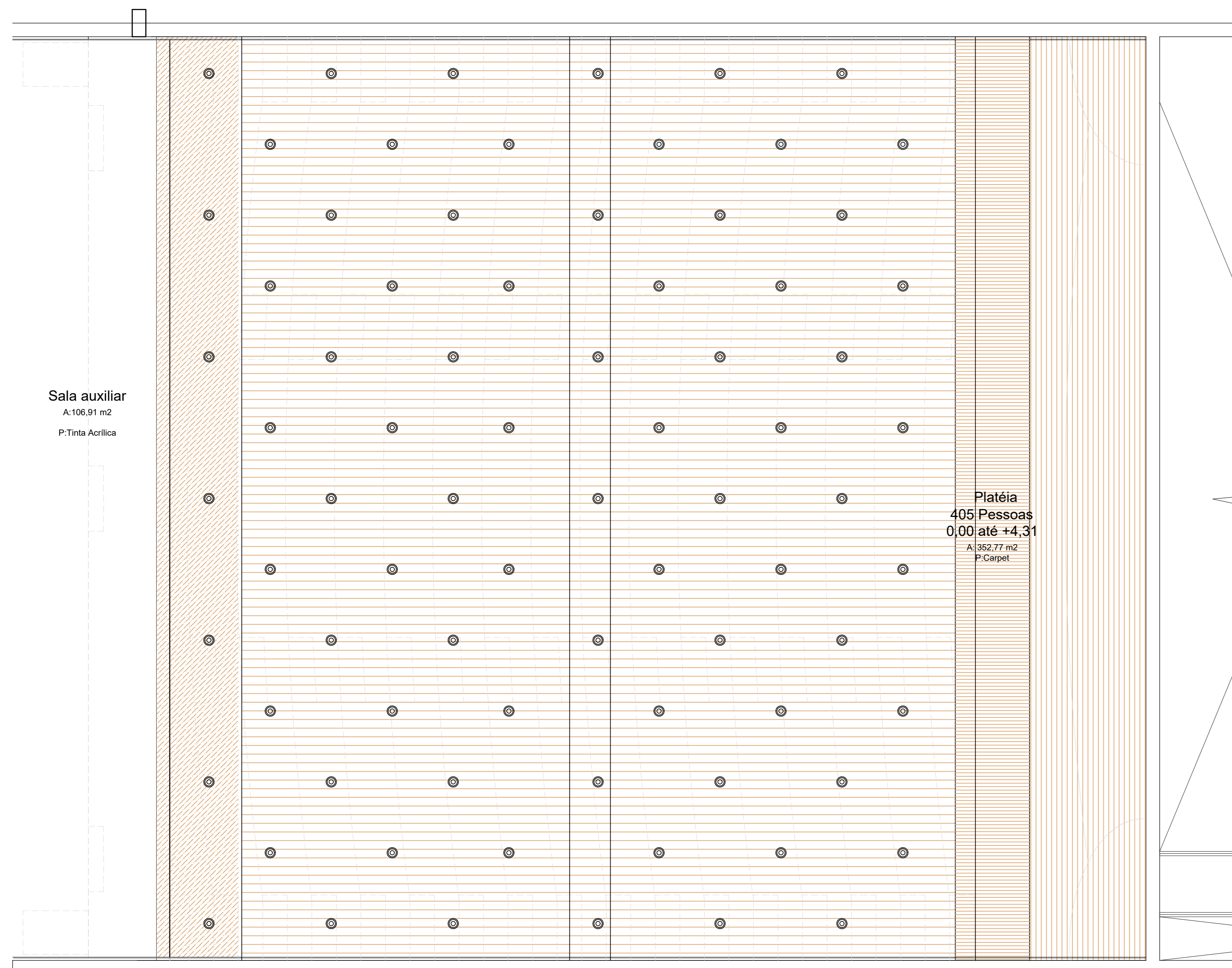
8 Paginação forro e iluminação platéia Escala 1:50
