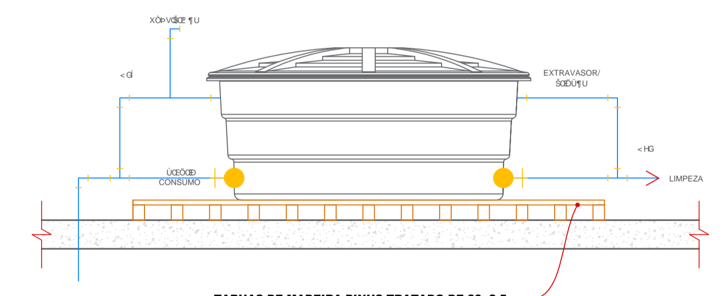
4 DET. CAIXA D'AGUA (BASE/LIMPEZA) ESCALA 1:25
