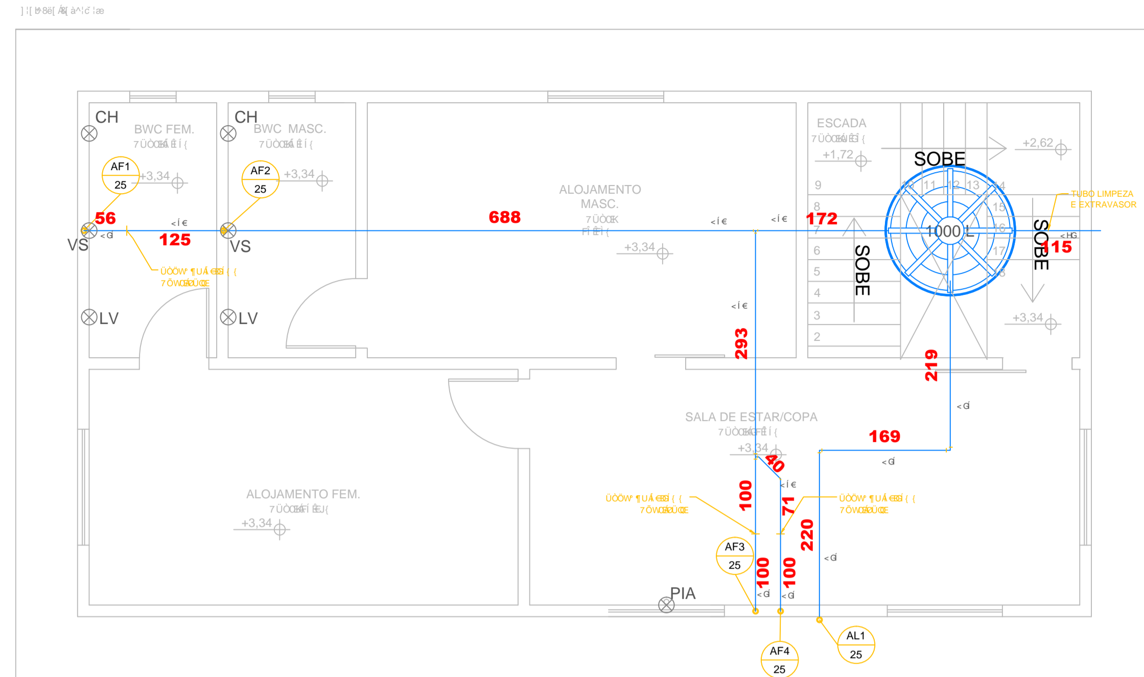
1 PLANTA BAIXA SUPERIOR - BARRILETE ESCALA 1:50
