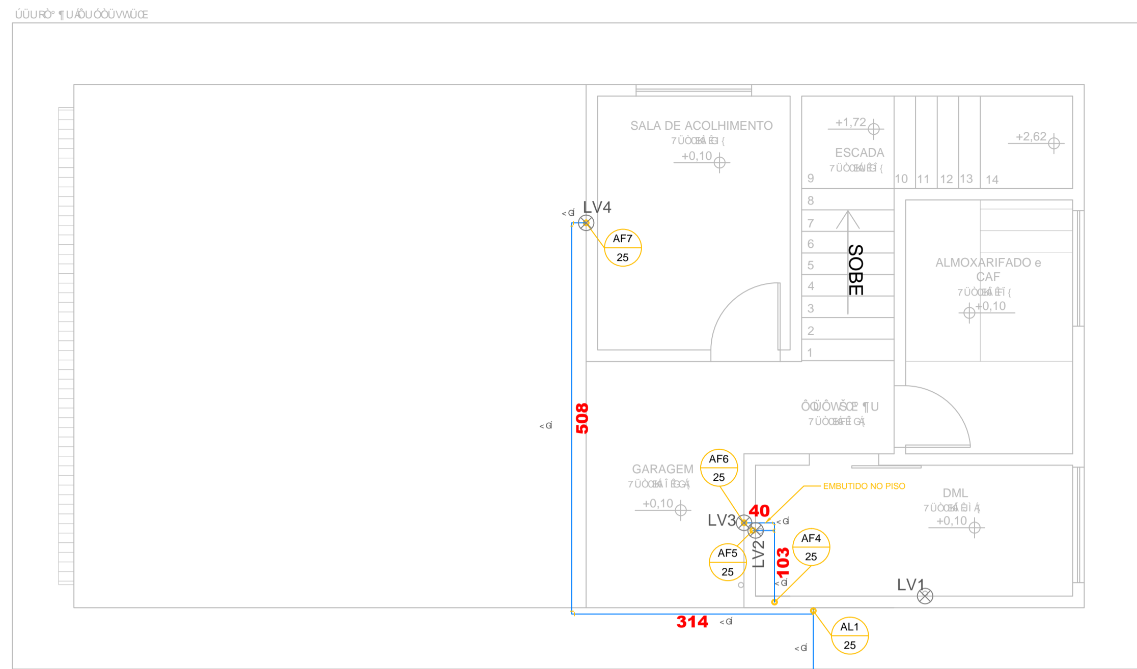
1 PLANTA BAIXA TERREO - BARRILETE ESCALA 1:50
