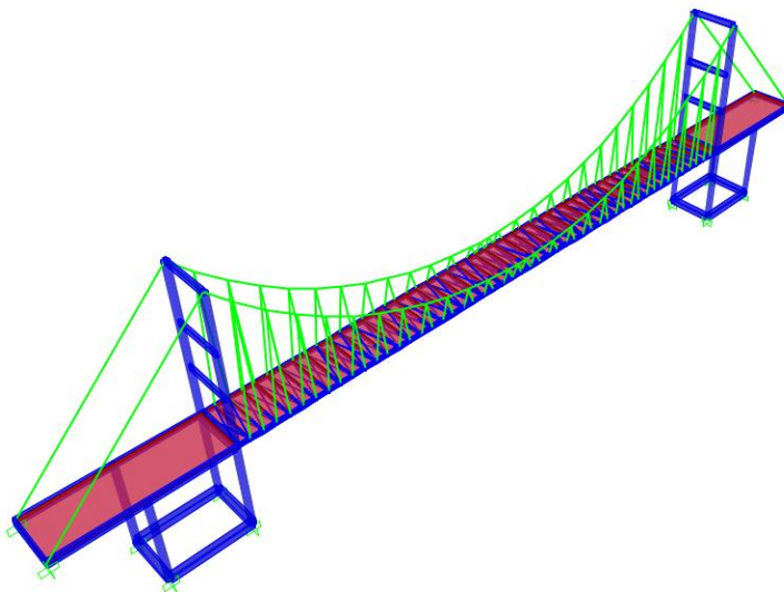
Figura 14 – Modelo estrutural
