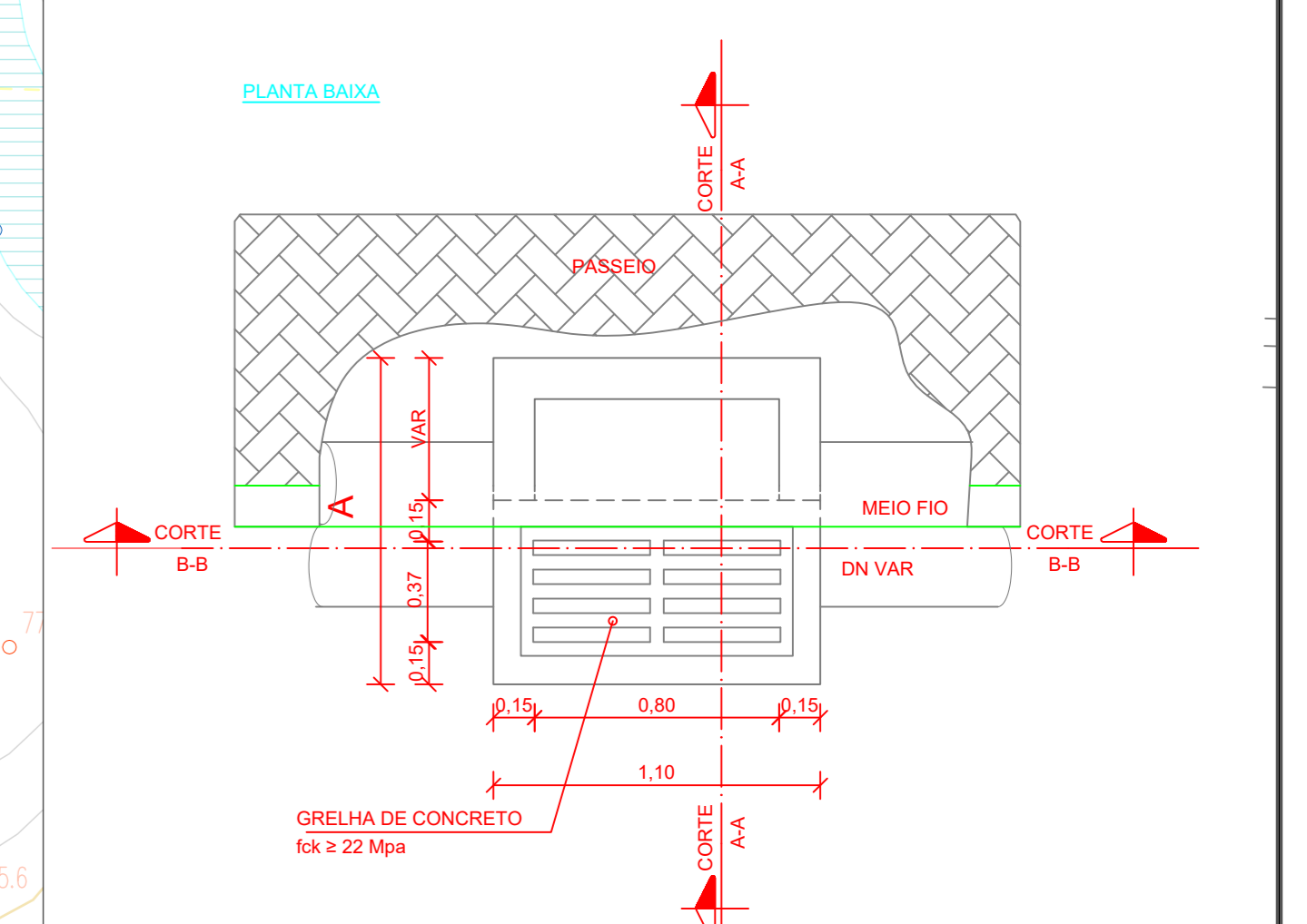
CAIXA COLETORA COM GRELHA DE CONCRETO (BOCA DE LULA)
